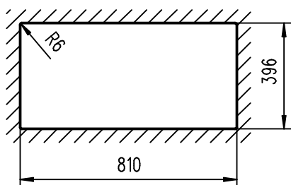
Ausschnitt Unterbau 1:20
